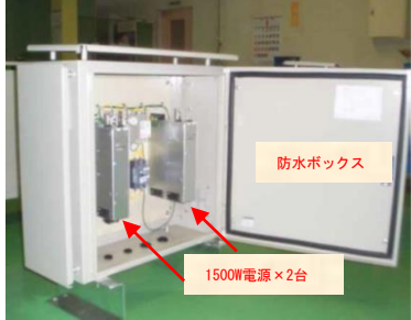
装置名：LEDサインシステム用電源装置
